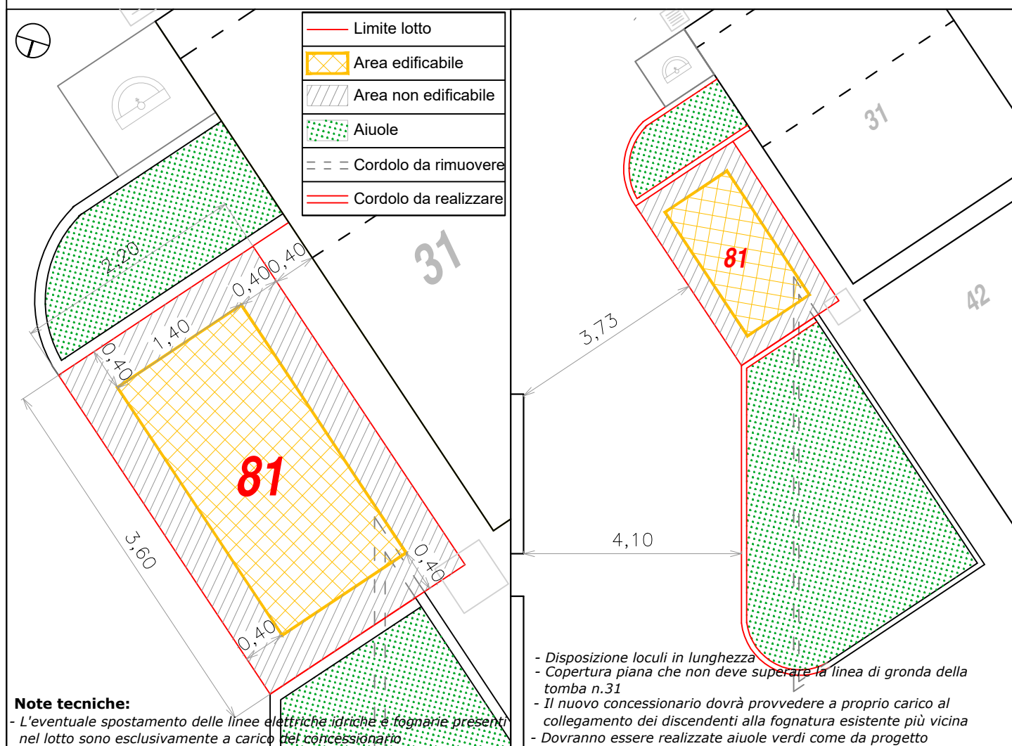
Planimetria Scala 1:50
